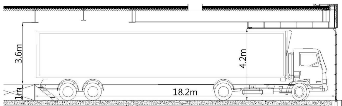
圖例 5.4 東碼頭卸貨口剖面圖
