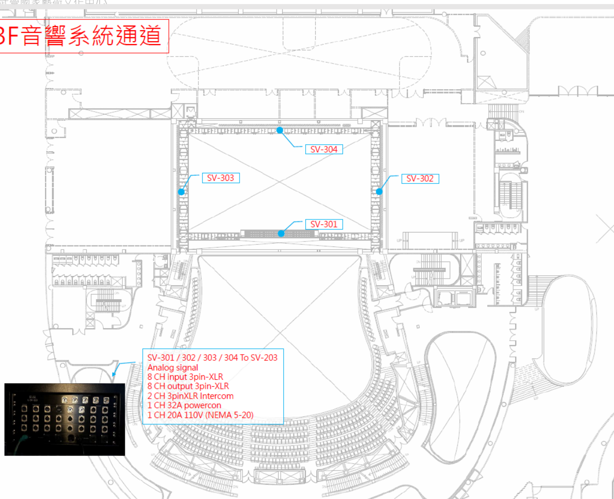
圖例 4-1.5 音響 3F 通道圖示
