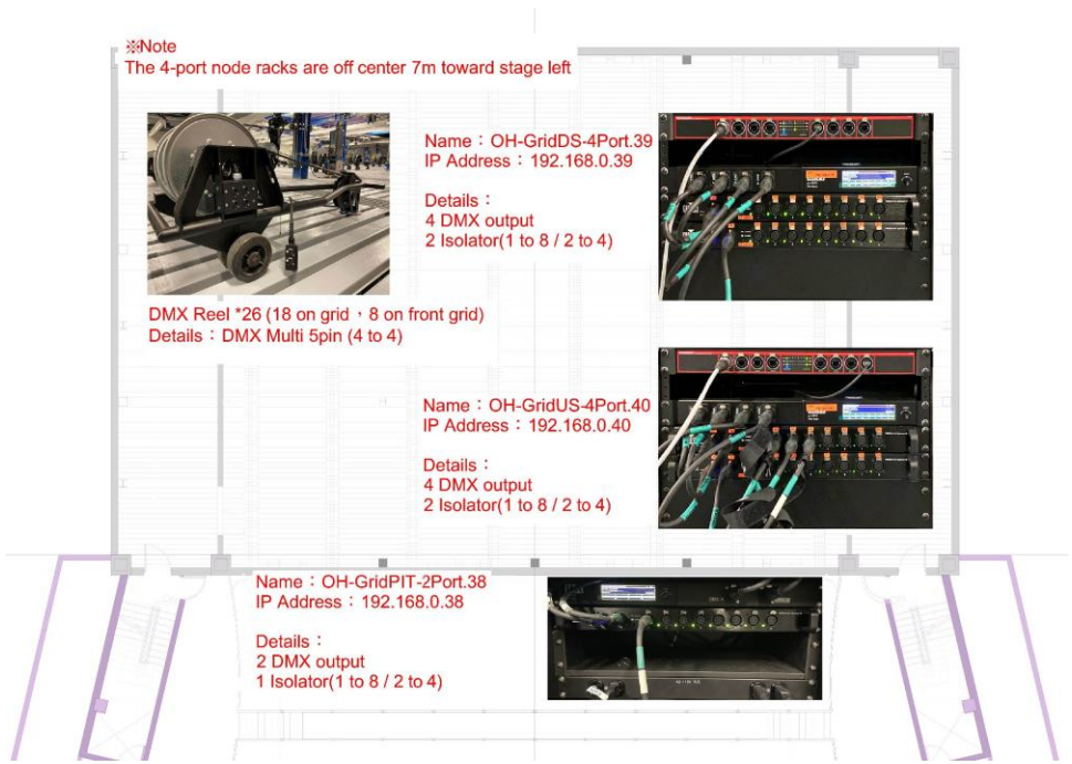
圖例 3.3.1- 頂棚區 Node 位置
