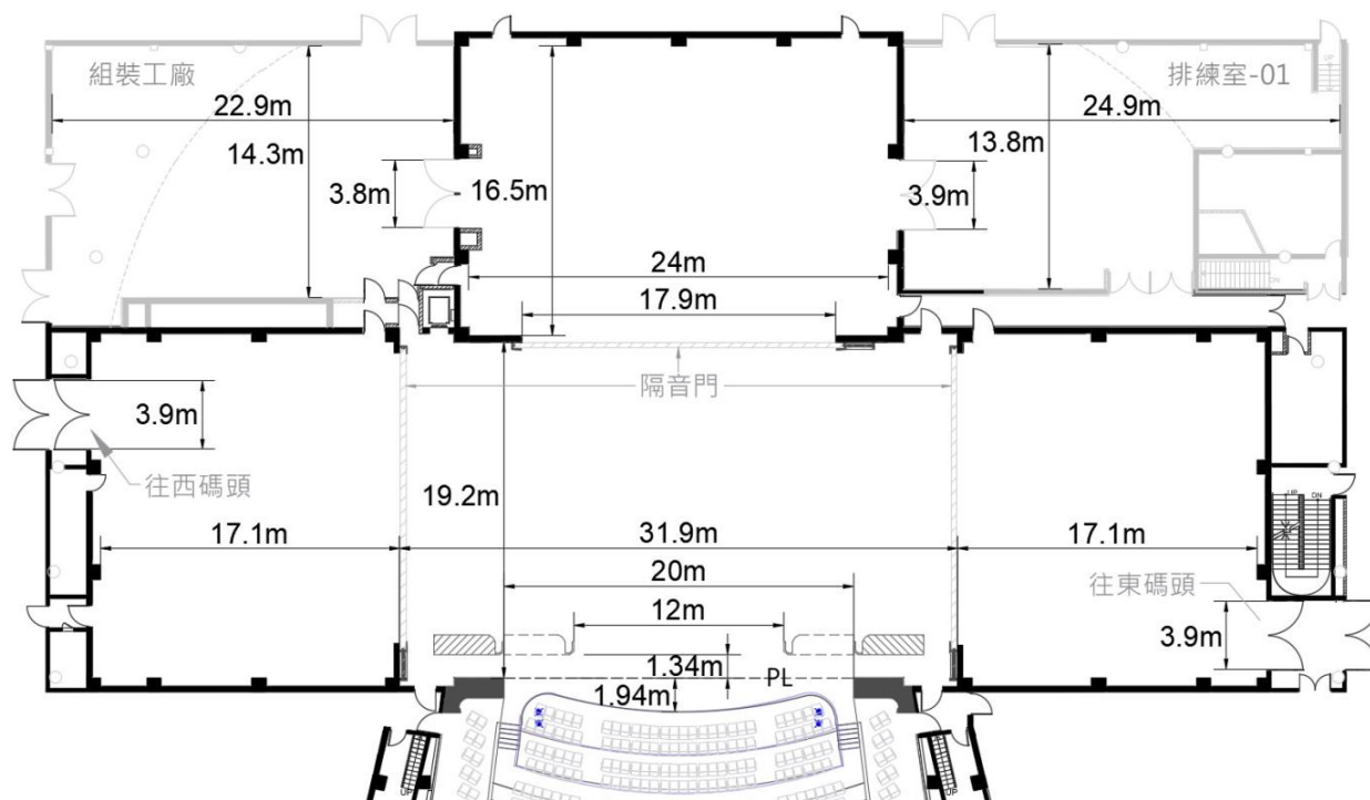
圖例 2.1.2-舞台平面圖
