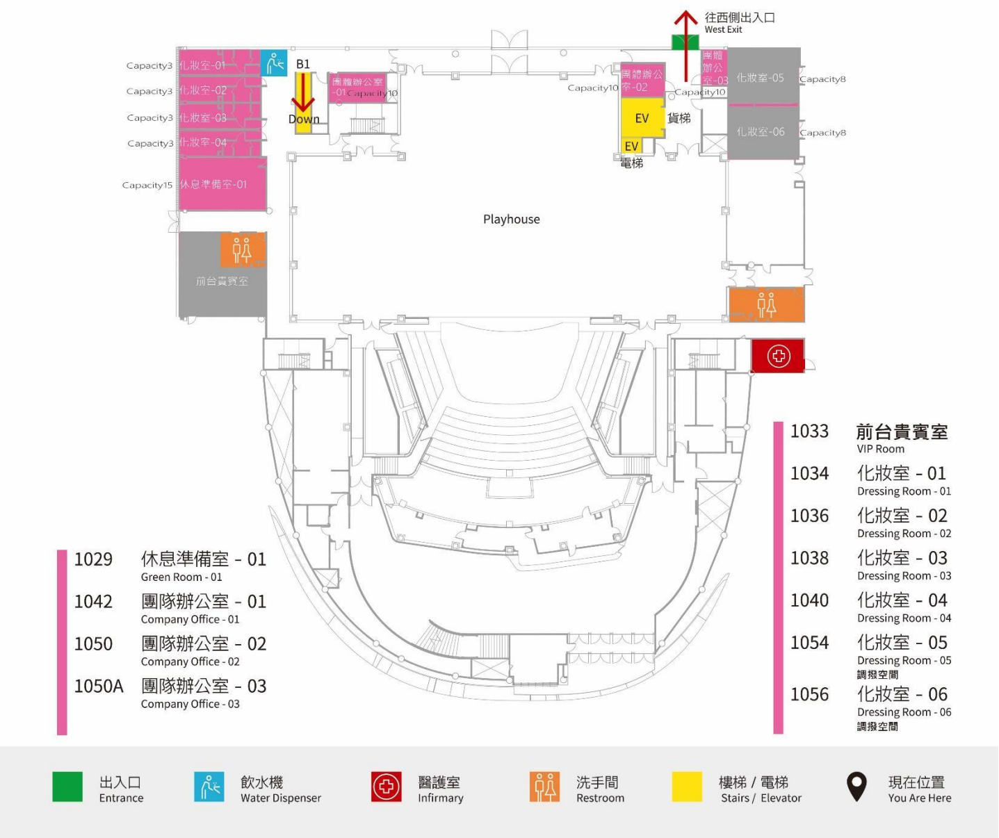
圖例 1.2-戲劇院一樓平面圖
