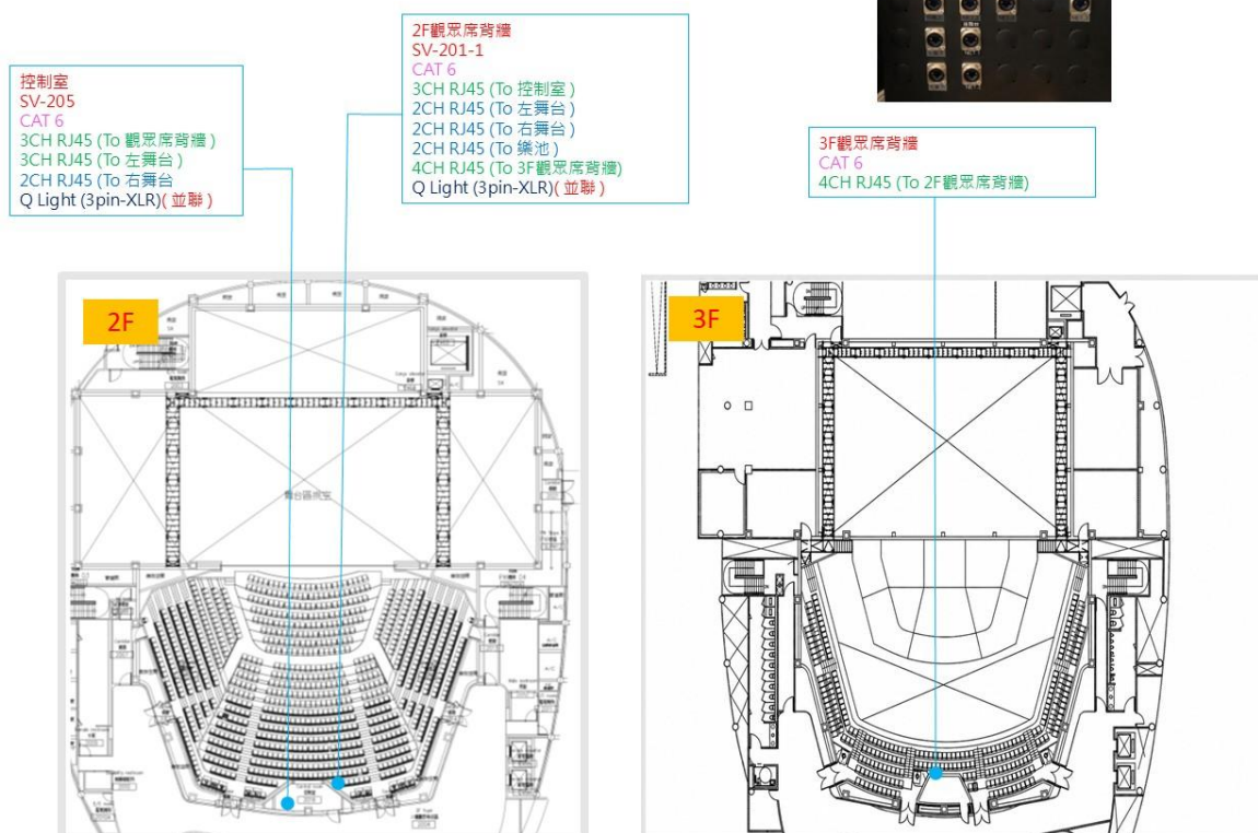
圖例 4-1.10 2F/3F RJ45 信號通道圖示
