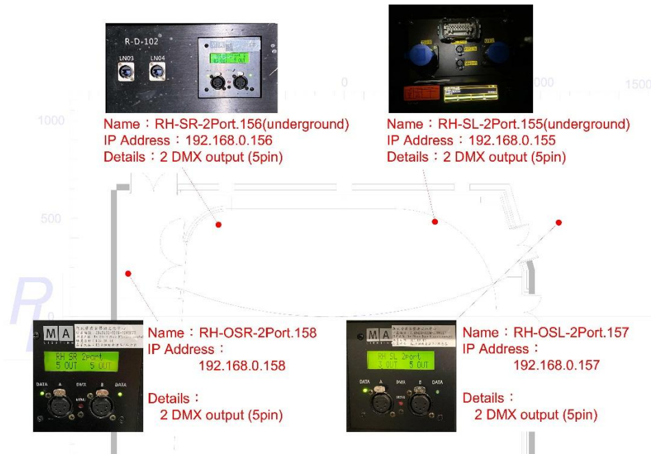
圖例 3.3.2- 舞台區 Node 位置圖
