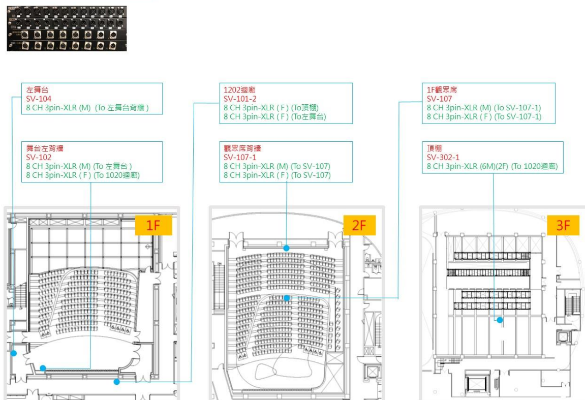
圖例 4-1.5 信號通道位置
