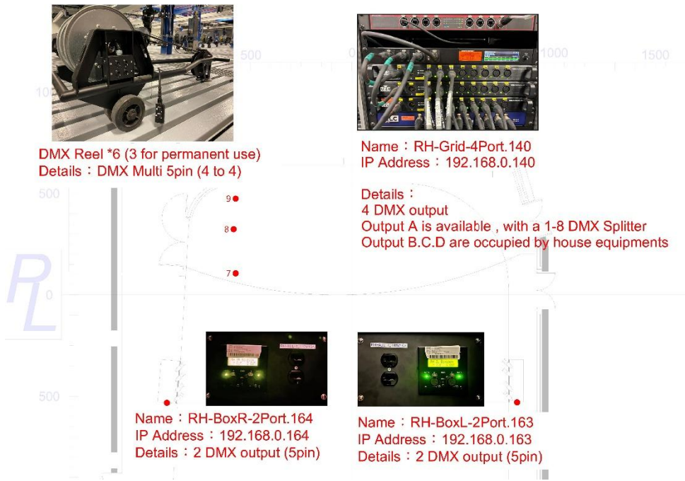
圖例 3.3.1- 頂棚及包廂區 Node 位置圖
