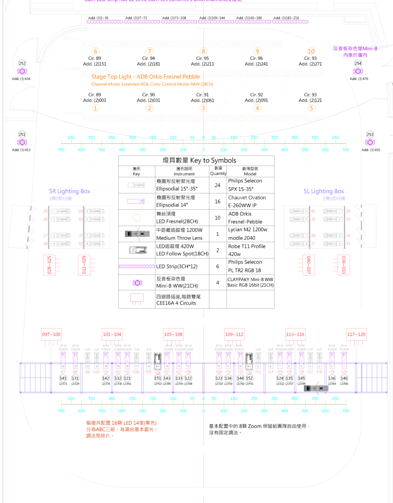
圖例 3.2.1- 燈光基本配置圖
