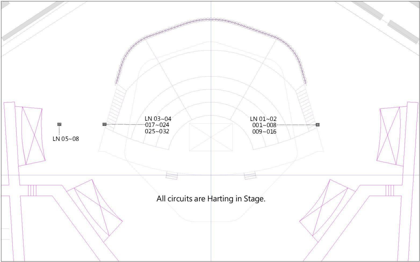
圖例 3.5.1.1- 舞台區燈光迴路配置
