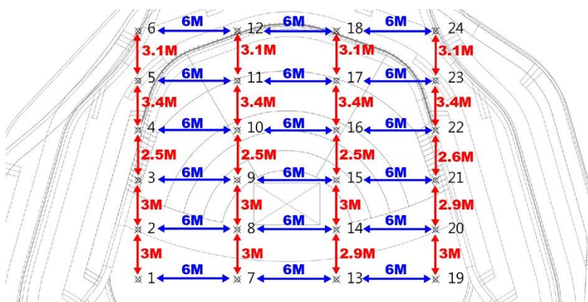
圖例 2.2 鍊條馬達位置圖
