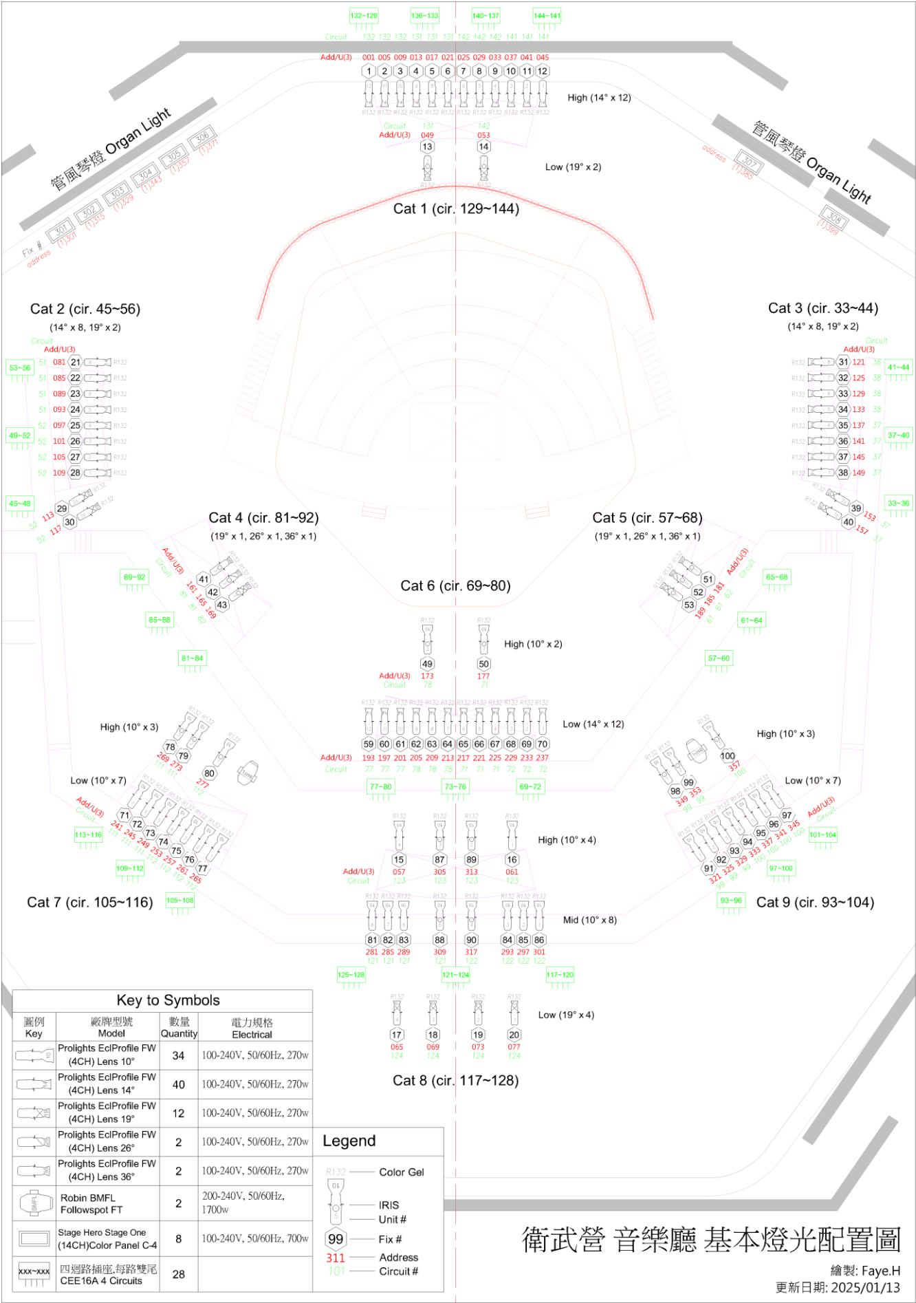
圖例 3.3.1- 燈光基本配置圖
