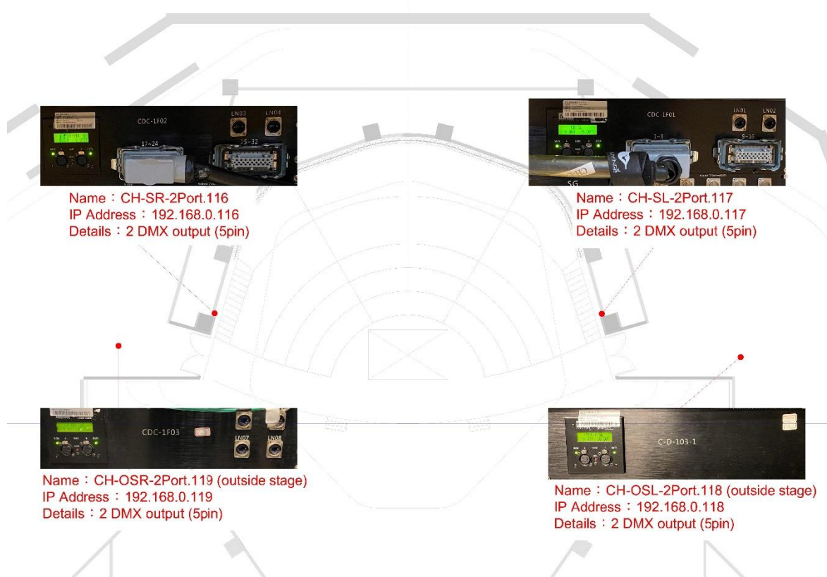
圖例 3.4.2- 舞台區 Node 位置圖
