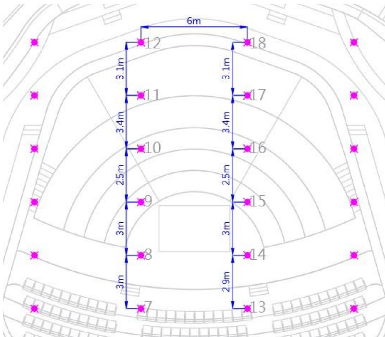
圖例 3.5.3- 可放迴路鍊條馬達出線孔
