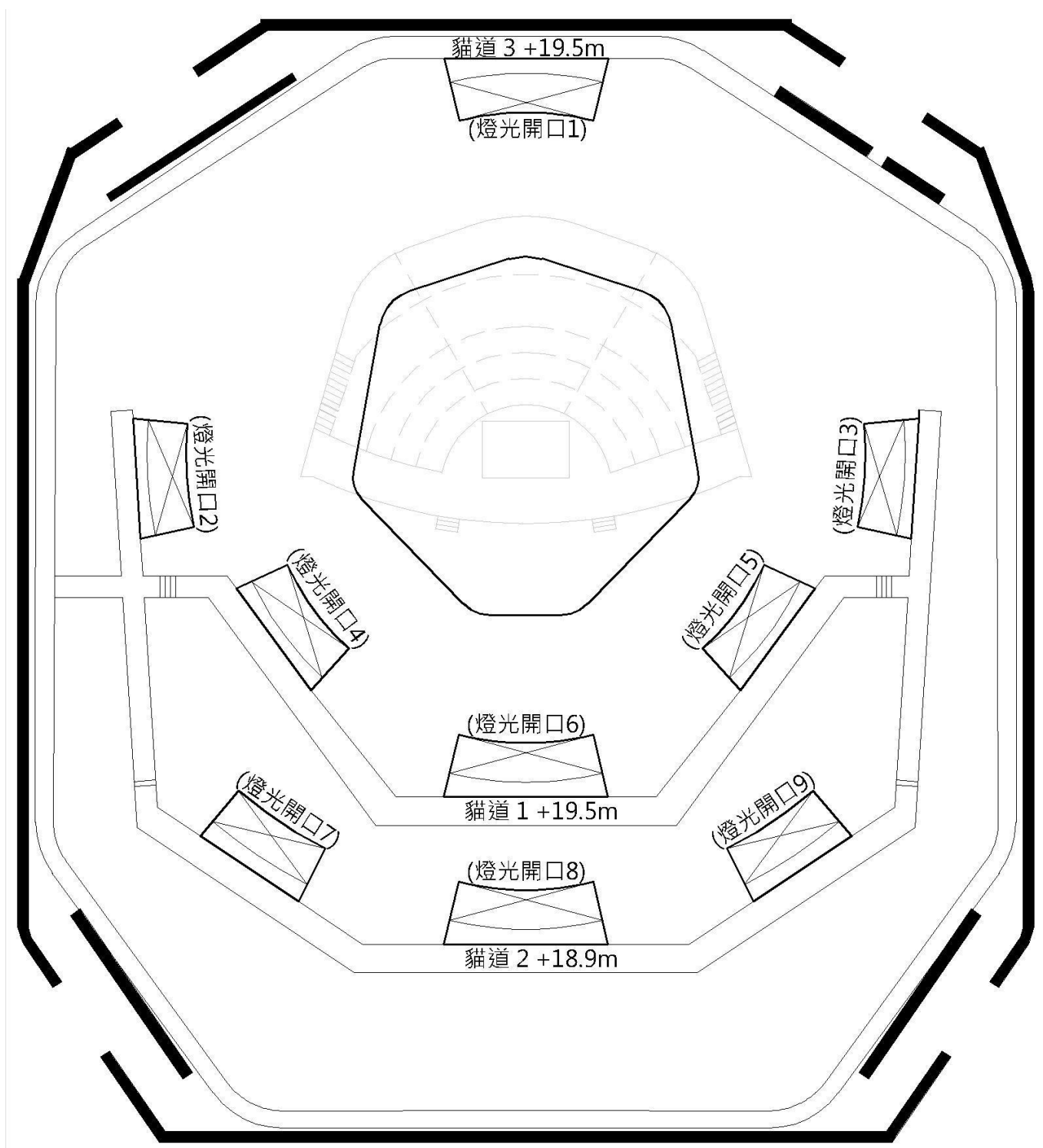
圖例 3.1 燈光開口位置平面圖
