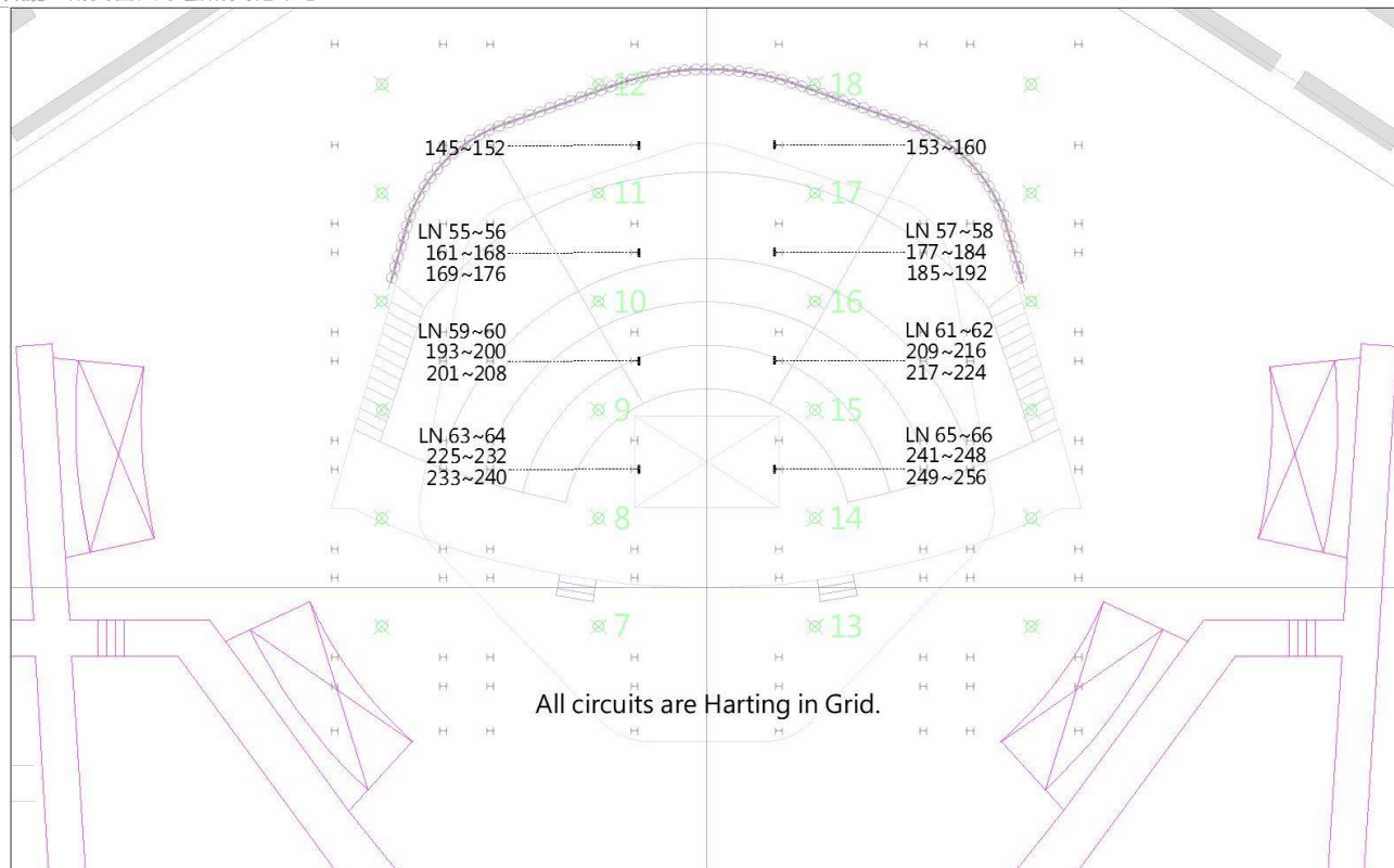
圖例 3.5.2.2- 舞台頂棚區燈光迴路配置
