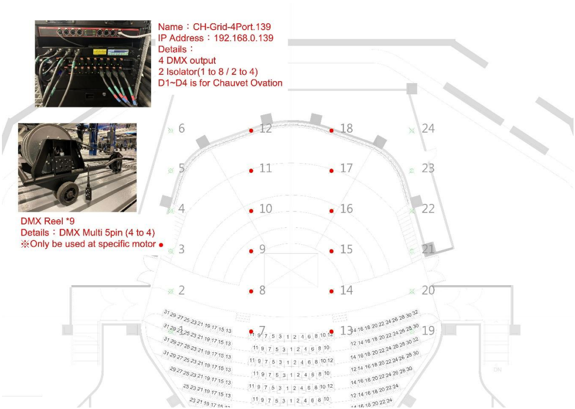
圖例 3.4.1- 頂棚區 Node 位置圖
