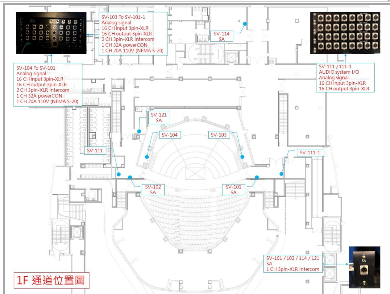
圖例 4-1.1 音響 1F 通道圖示
