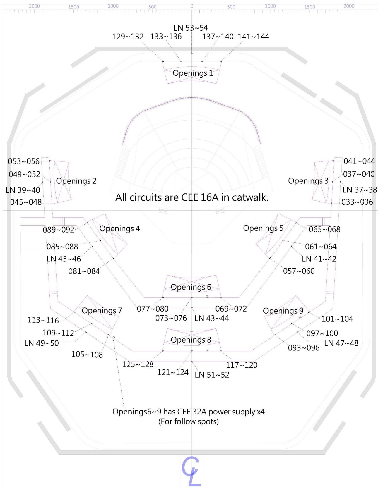
圖例 3.5.2.1- 外區燈光迴路配置
