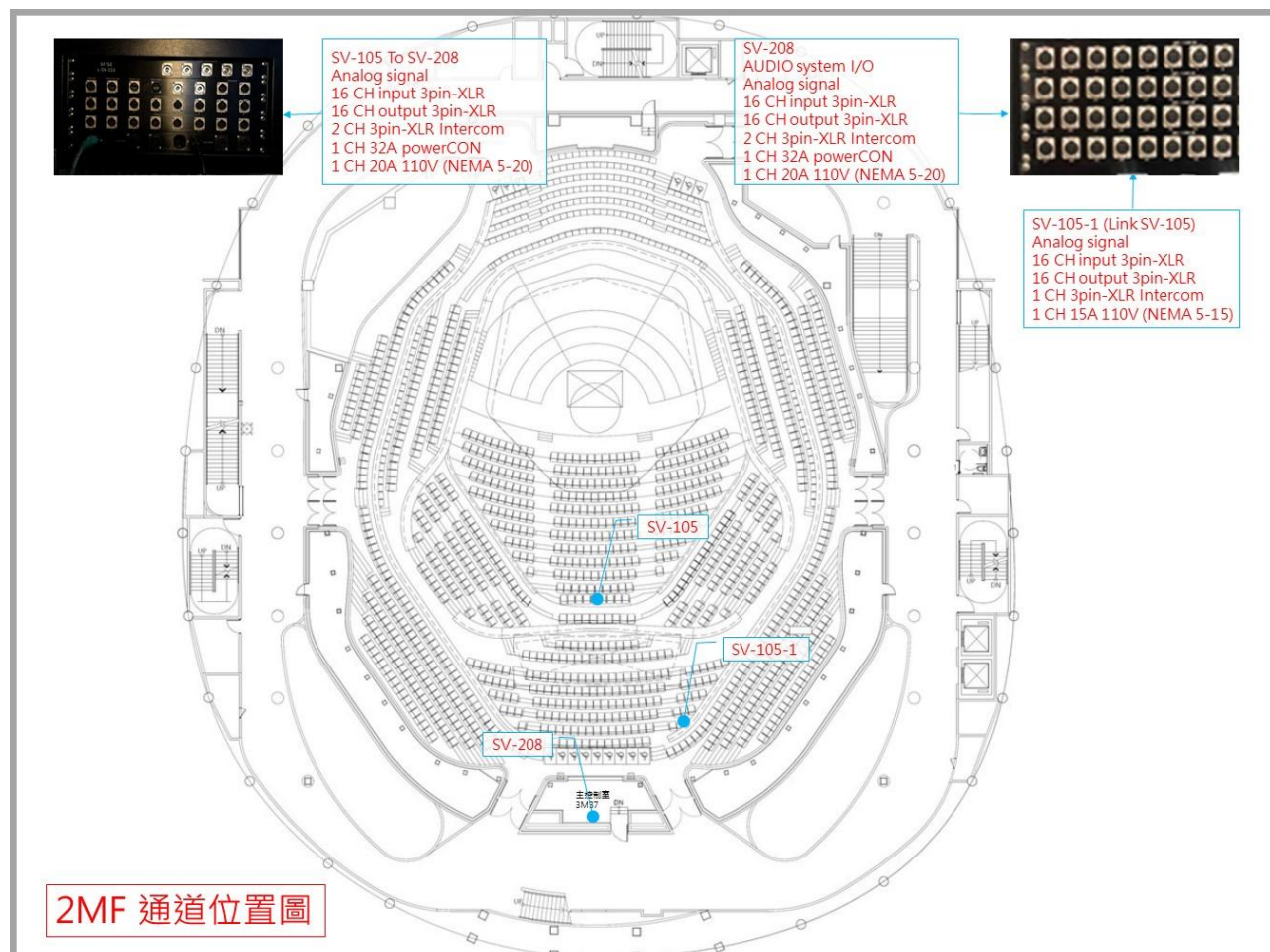
圖例 4-1.2 音響 2MF 通道圖示
