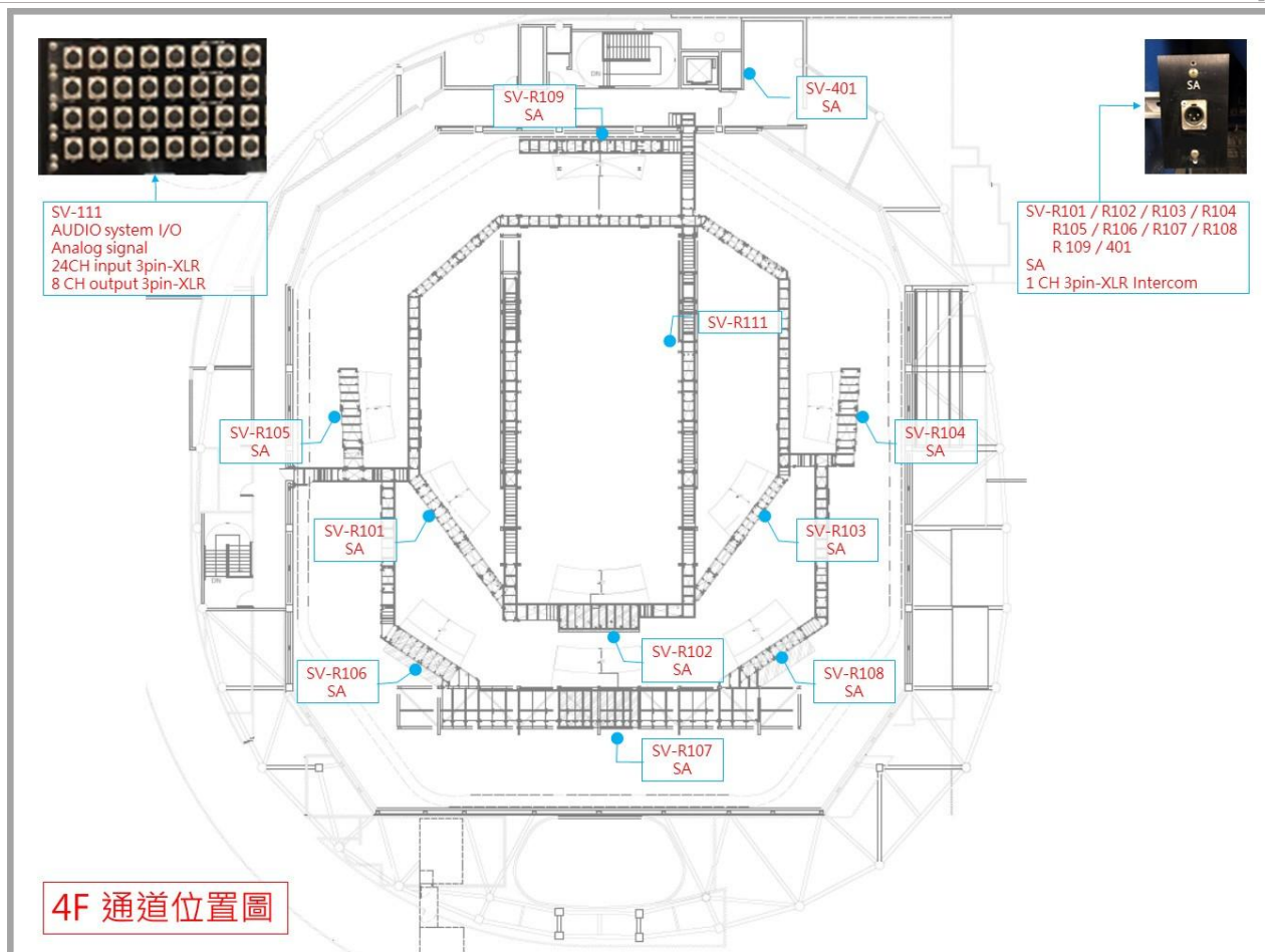
圖例 4-1.3 音響 4F 通道圖示
