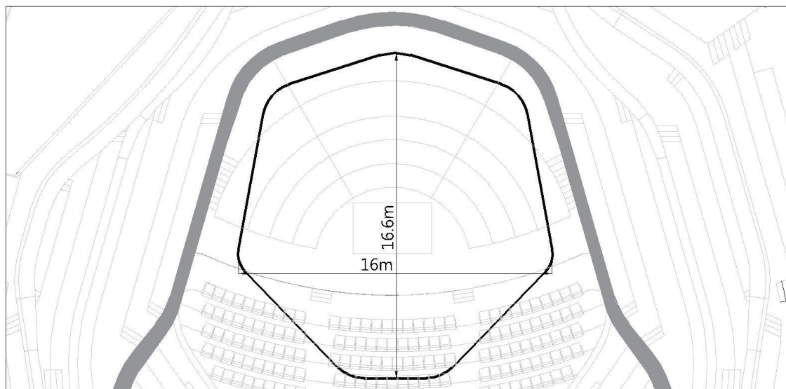
圖例 2.4-音響反射板位置圖
