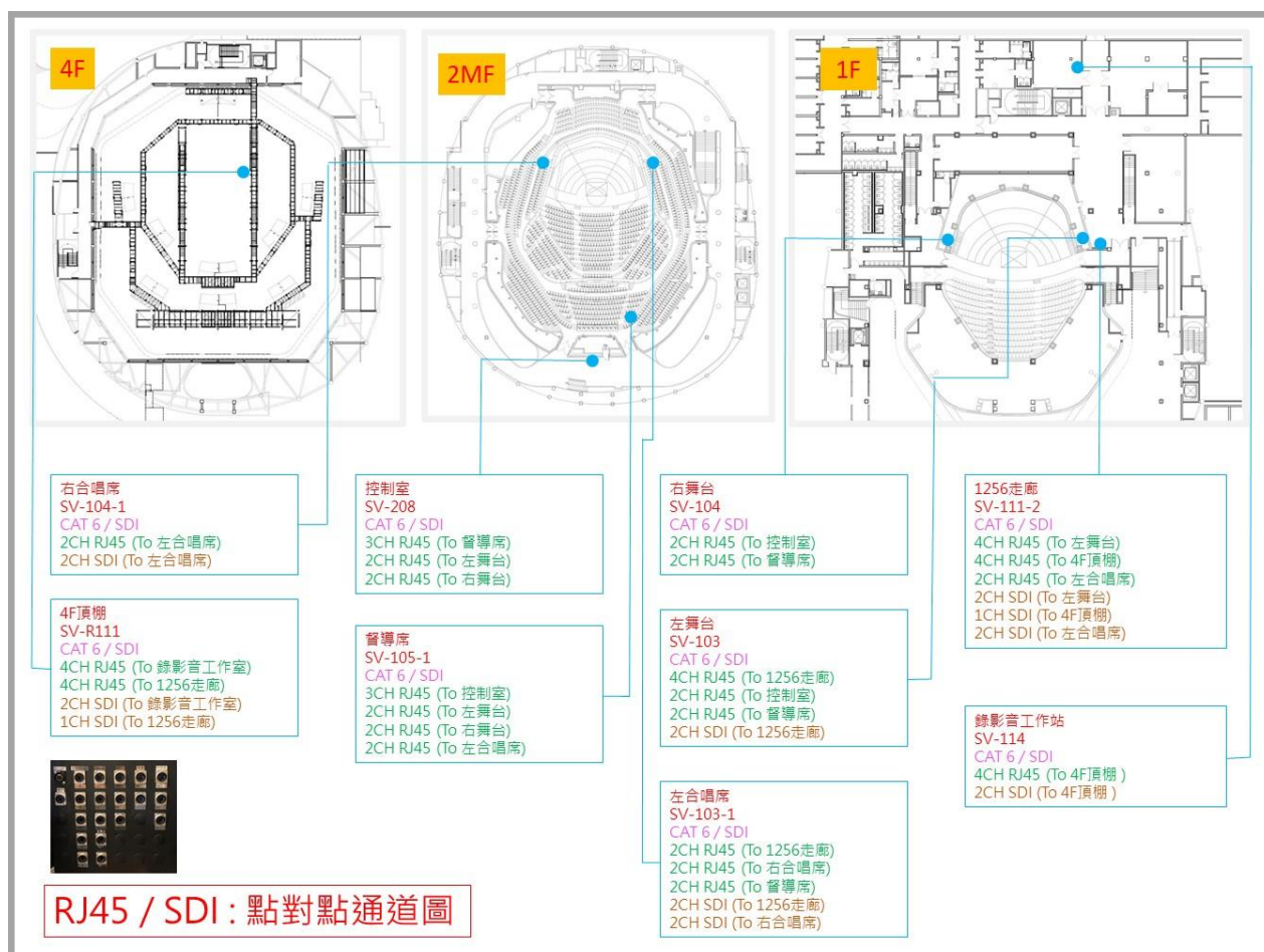
圖例 4-1.6 RJ45 / SDI 通道圖示
