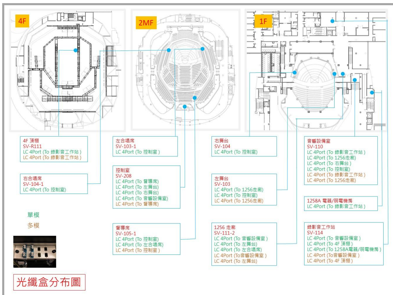
圖例 4-1.4 光纖通道圖示
