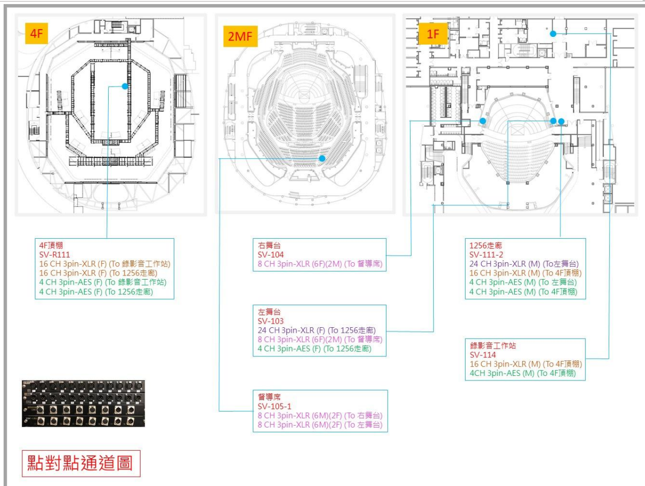
圖例 4-1.5 信號通道圖示
