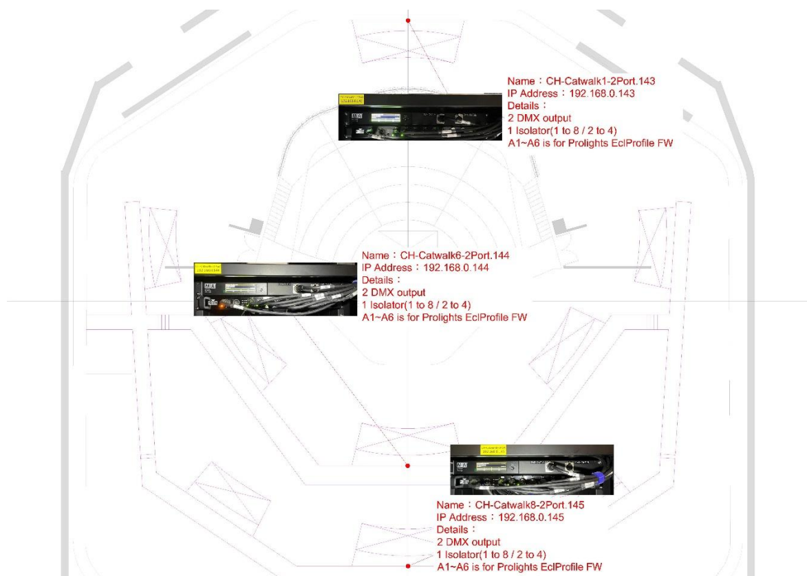
圖例 3.4.3- 貓道區 Node 位置圖
