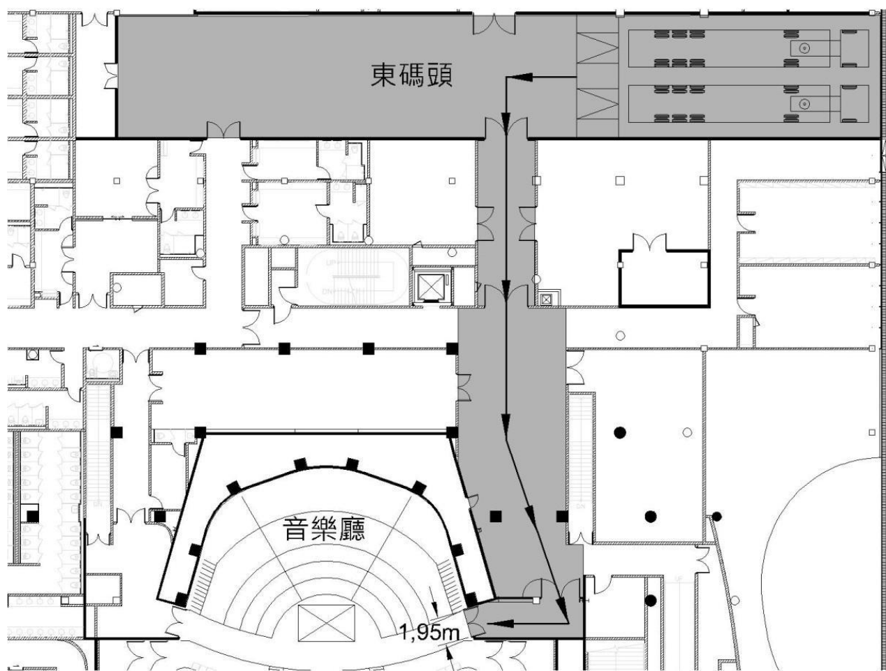
圖例 5.3 卸貨動線
