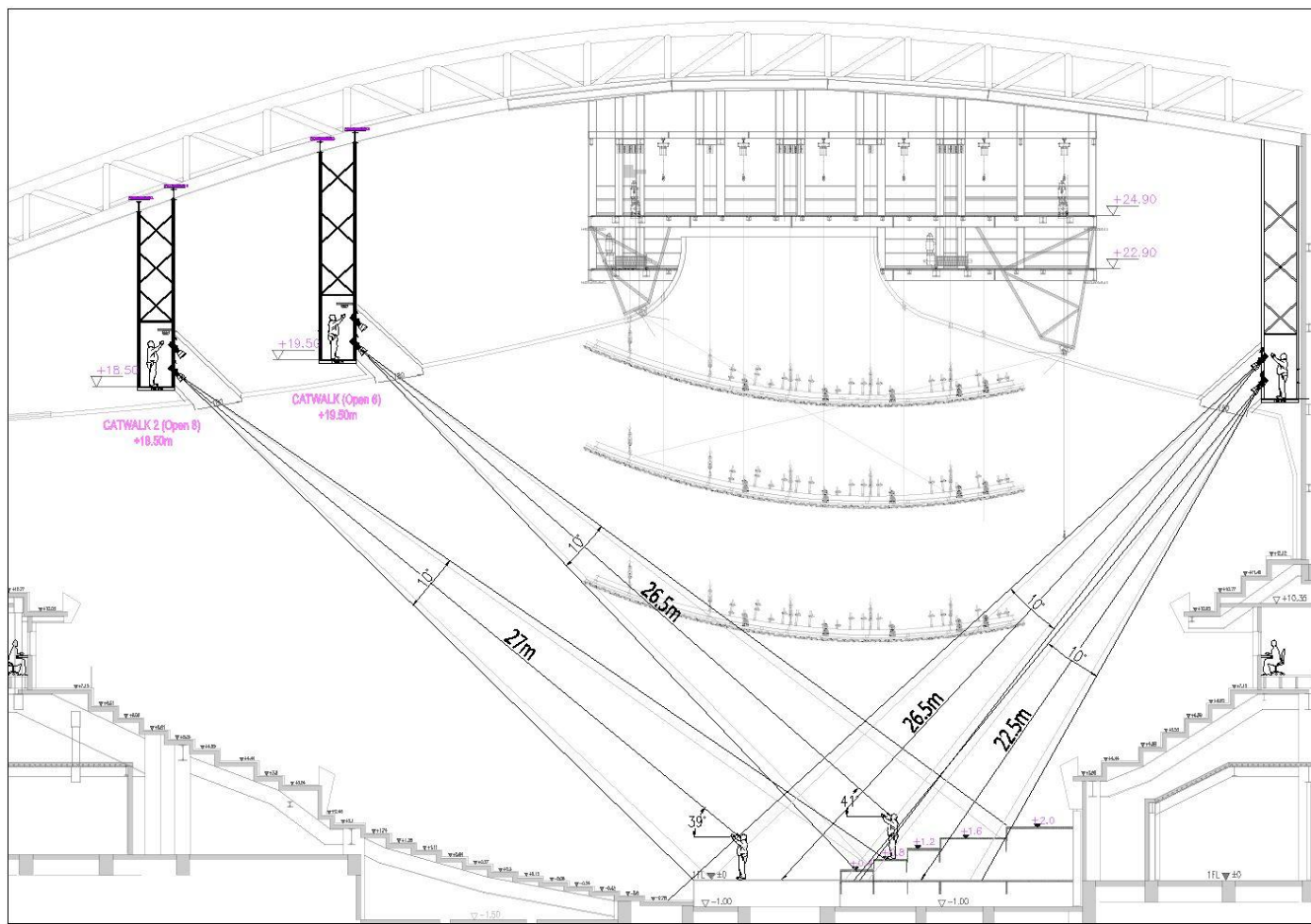
圖例 3.3.2- 燈光剖面圖
